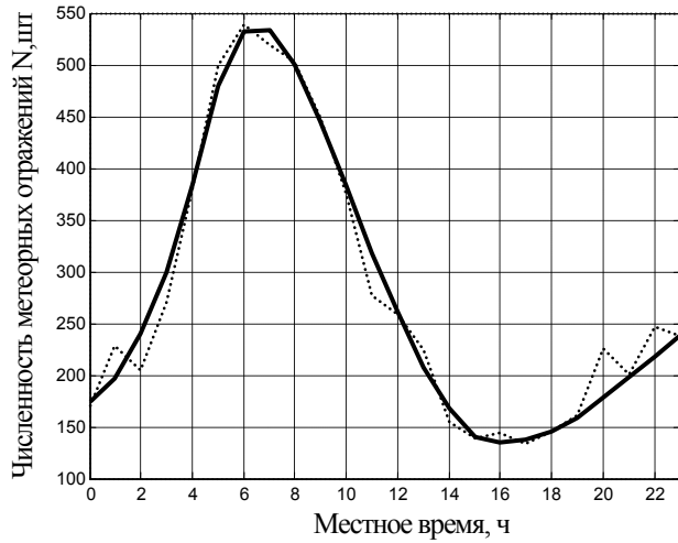
Рис. 11. Усредненный суточный ход численности отражений от метеоров потока Гемениды
