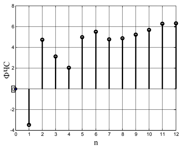
Рис. 14. АЧС и ФЧС суточного хода численности метеоров потока Гемениды
