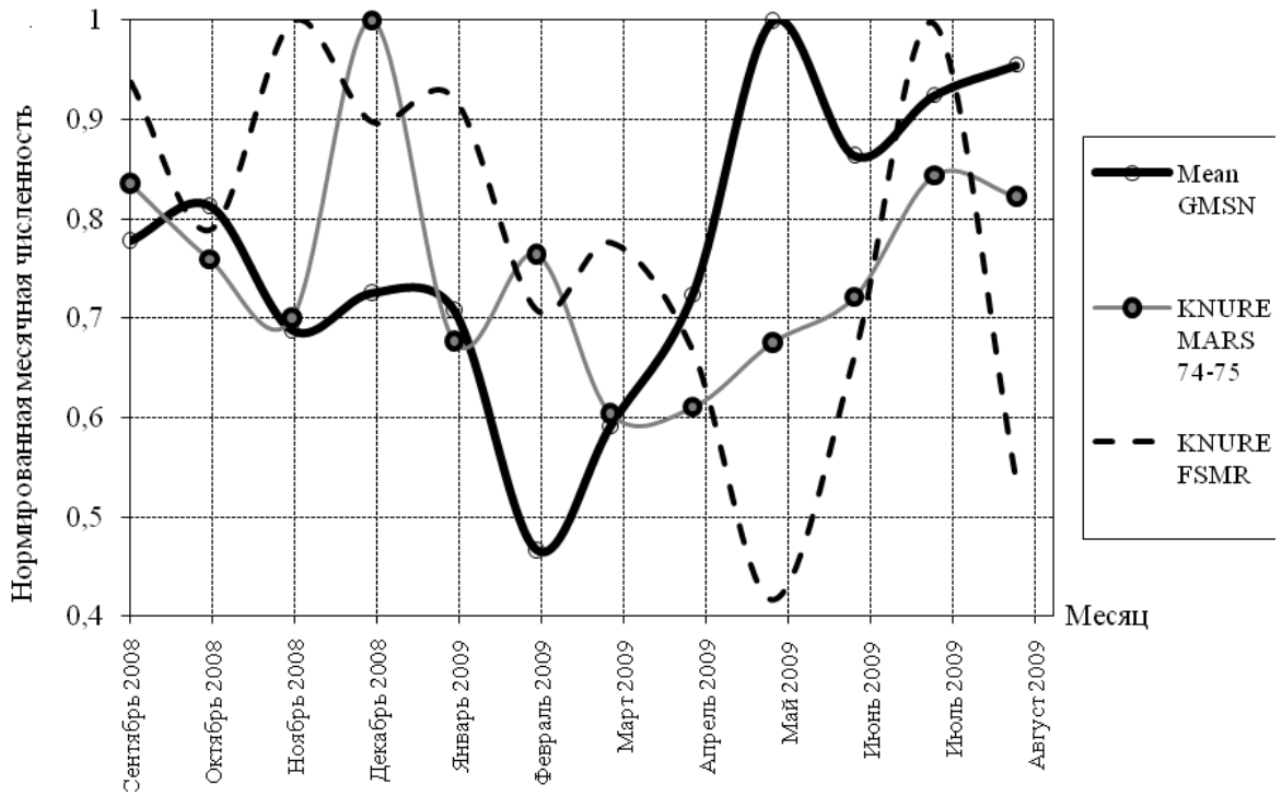
Рис. 8. Сезонная вариация среднемесячной численности метеорных отражений
