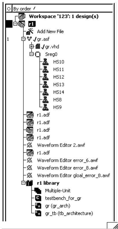
Рис. 3. Структура файлов комплекса
