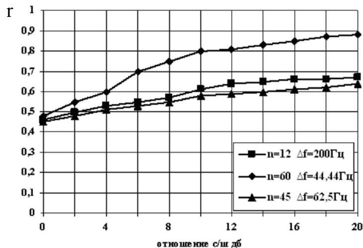
Рис. 1. Результати статистичних випробувань оцінки величини довірительного інтервала в залежності від відношення сигнал/шум
