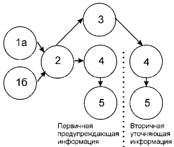
Рис. 1. Схема інформування населення: 1а – очевидець аварії; 1б – автоматична сигналізація; 2 – оперативний дежурний МНС; 3 – аналітичний центр; 4 – сотовий оператор, що виконує розсилку повідомлень; 5 – абоненти мережі, що знаходяться в ураженій місцевості
