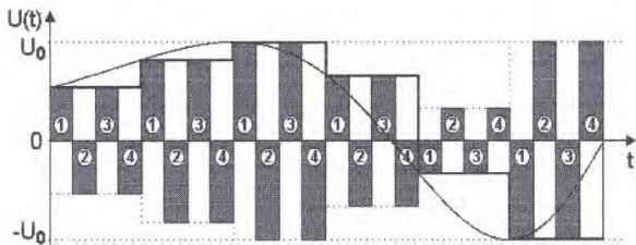
Рис. 3. Сигнал на выходе коммутатора при P = 4
