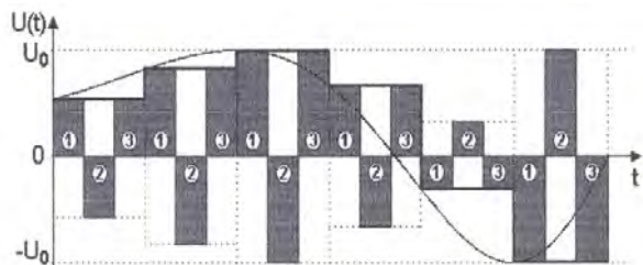
Рис. 4. Сигнал на выходе коммутатора при P = 3
