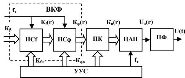
Рис. 1. Обобщенная структурная схема цифрового синтезатора сигналов
