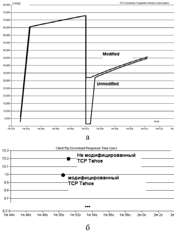
Рис. 4. Залежність розміру перегруженого вікна (а) і часу передачі пакета в установленному з'єднанні (б) від часу моделювання для стандартної версії протоколу TCP Tahoe і його пропозованої модифікації
