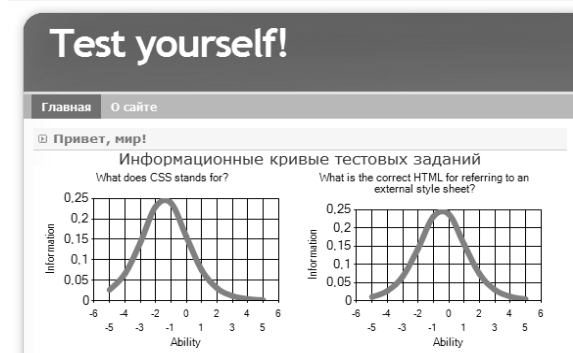
Рис. 5. Пример построения информационных кривых тестовых заданий
