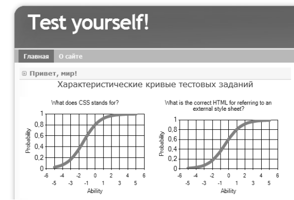
Рис. 5. Пример построение характеристических кривых тестовых заданий
