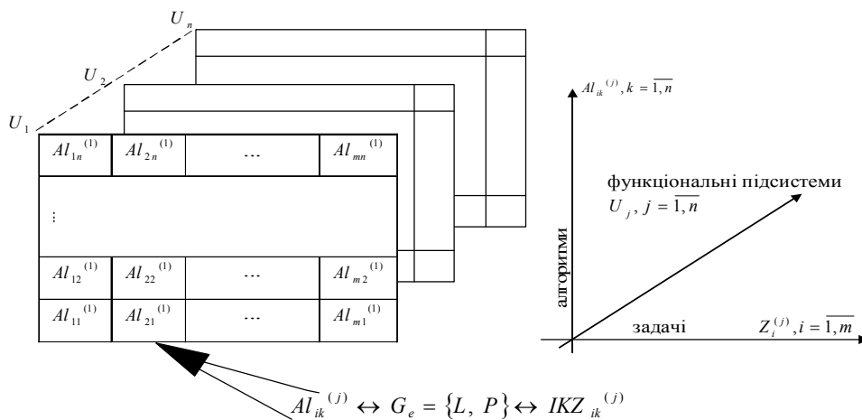
Рис. 4. Багатомірне представлення AI \subset Z \subset U
