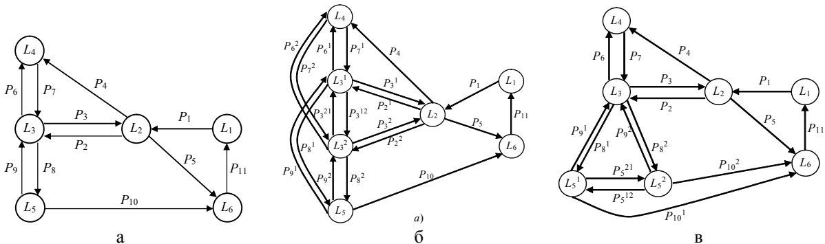
Рис. 6. Граф найпростішого (а) та ускладненого (б, в) інформаційного контуру
