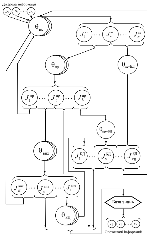
Рис. 3. Графове представлення МОІР вузлової ІСУ
