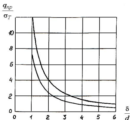
Рис. 7. Зависимость отношения давления пробивки к пределу текучести материала от относительной величины отверстия
