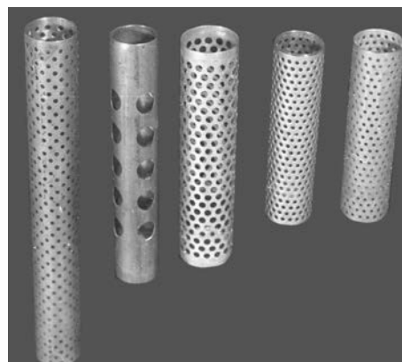
Рис. 2. Образцы перфорированных трубок, изготовленные методом ГДШ на пресс-пушках с располагаемой энергией до 20 кДж
