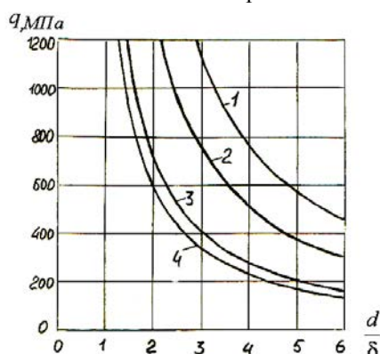
Рис. 8. Зависимость требуемого давления пробивки для различных материалов: 1 – сталь 20, нагартованная; 2 – сталь 20, отожженная; 3 – латунь Л62; 4 – алюминиевый сплав Д16АМ
