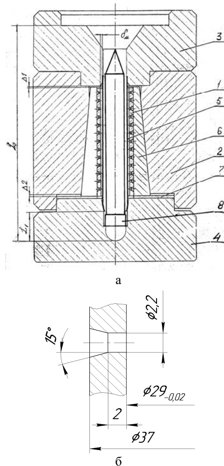
Рис. 14. Конструктивная схема оснастки с профилированными отверстиями матрицы и разрезной обоймой (а):
