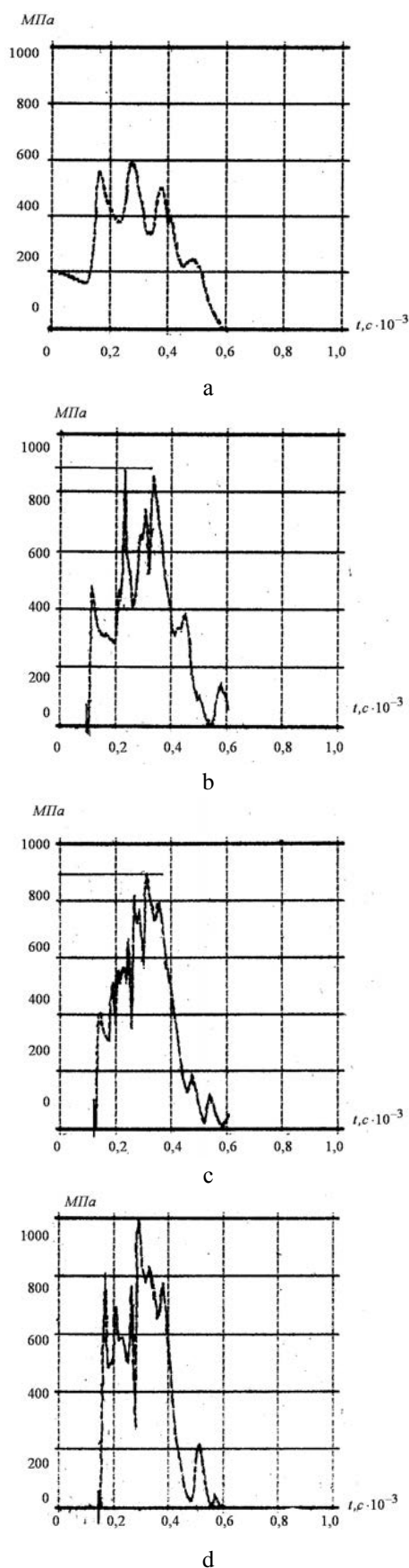
Рис. 12. Динамика развития волны давления жидкости внутри полости заготовки: а – непосредственно под днищем снаряда; б – в верхней части заготовки; с – в средней части заготовки; д – в нижней части заготовки
