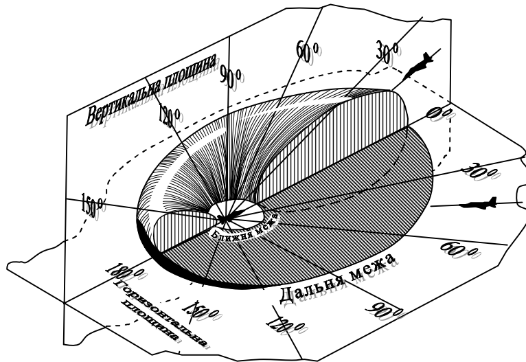
Рис. 1. Область безпеки повітряного судна при виконанні маршрутного польоту
