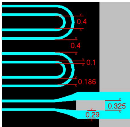
Рис. 1. Топология изготовления копланарной линии передач
