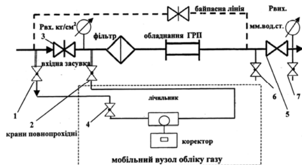
Рис. 3. Схема підключення переносного комплексу в ГРП
