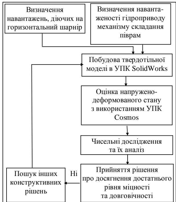
Рис. 4. Послідовність оцінювання навантаженості корпусу шарнірного зчленування
