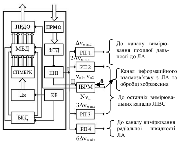
Рис. 1. Загальна схема структури приймально-передавальної частки каналів ЛВС з ЧЧМ
