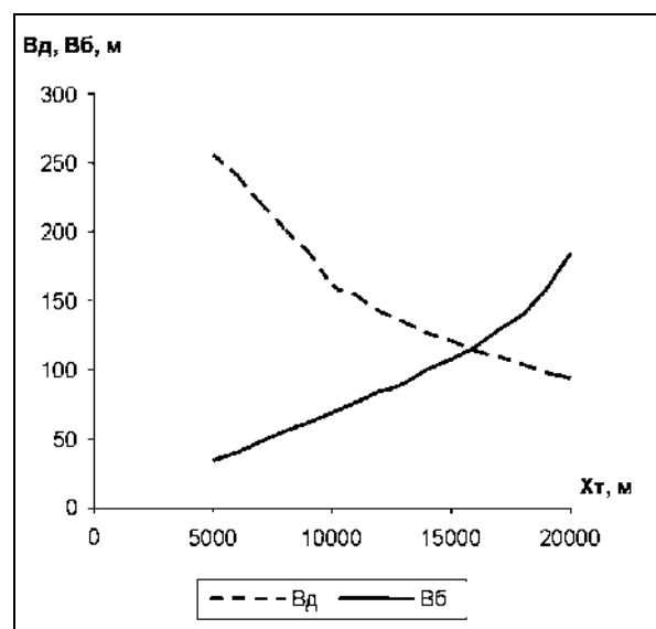
Рис. 2. Графіки характеристик розсіювання V\delta , V\delta_0 залежно від дальності стрільби
