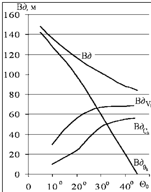
Рис. 1 Складові сумарного розсіювання по дальності для оперених реактивних снарядів
