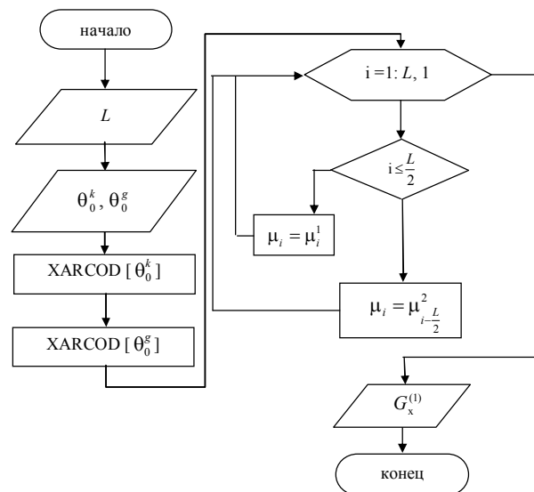
Рис. 3. Алгоритм формирования составной последовательности с использованием усовершенствованного метода
