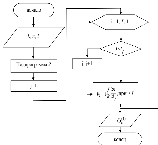
Рис. 2. Алгоритм формирования составной последовательности по правилу присоединения
