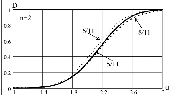
Рис. 3. Показники якості виявлення ПЦ вторинним каналом СВЦ
