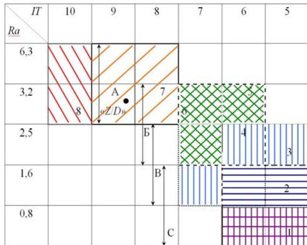
Рис. 3. Структура матрицы данных для выбора методов механической обработки наружных цилиндрических поверхностей деталей с учетом качества IT и шероховатости поверхности Ra (области А, Б, С и Д)
