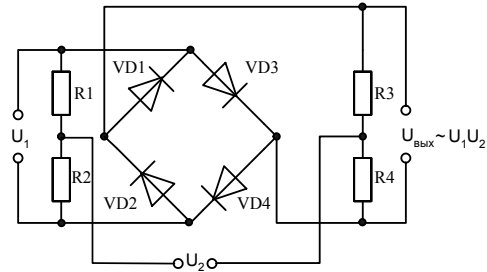
Рис. 2. Кольцевая балансная схема
