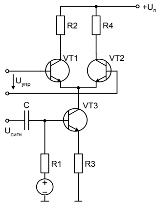
Рис. 6. Схема ДУ
