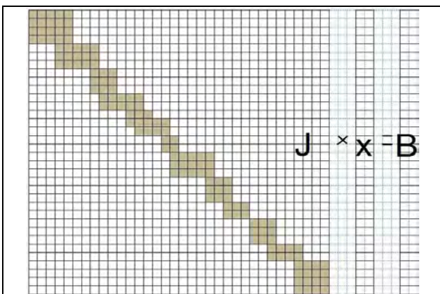
Рис. 3. Структура математической задачи, которая решается при моделировании ГТС
