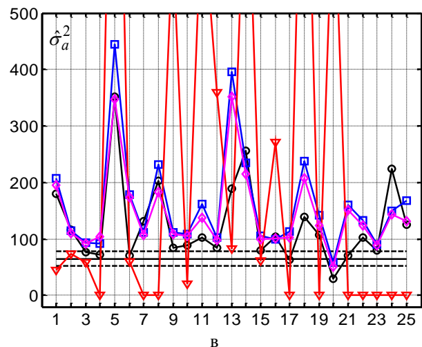
Рис. 2. Сравнительный анализ результатов оценивания дисперсии коррелированного шума ( \sigma_a^2 = 65 ) на изображениях из базы TID2008 (красная компонента): а – исходные изображения, б, в – изображения, прореженные в 2 и 3 раза соответственно
