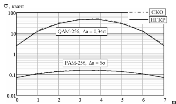
Рис. 2. СКО сигналов N-OFDM на основе ПХ с различными видами модуляций несущих при равном частотном уплотнении ( \xi_p = 2,71 )
