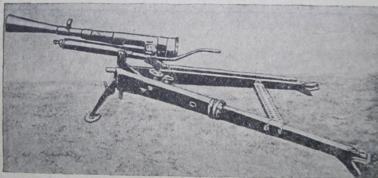
Рис. 59. 37-мм пехотная пушка обр. 1916 г.
