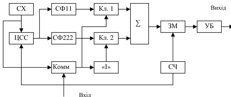
Рис. 1. Структурна схема передавальної сторони
