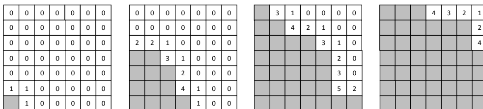
Рис. 2. Розподіл параметра SP в різні моменти часу моделювання
