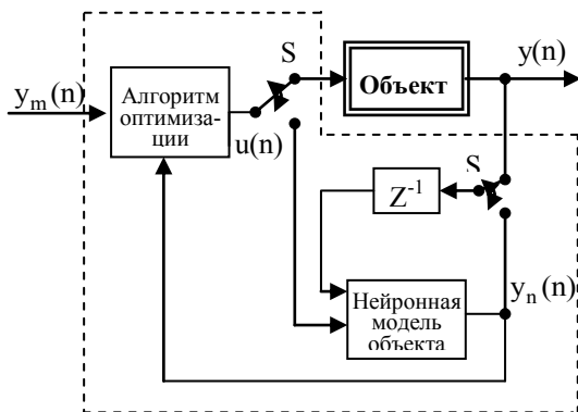
Рис. 3. Схема системи нейруправління з прогнозом
