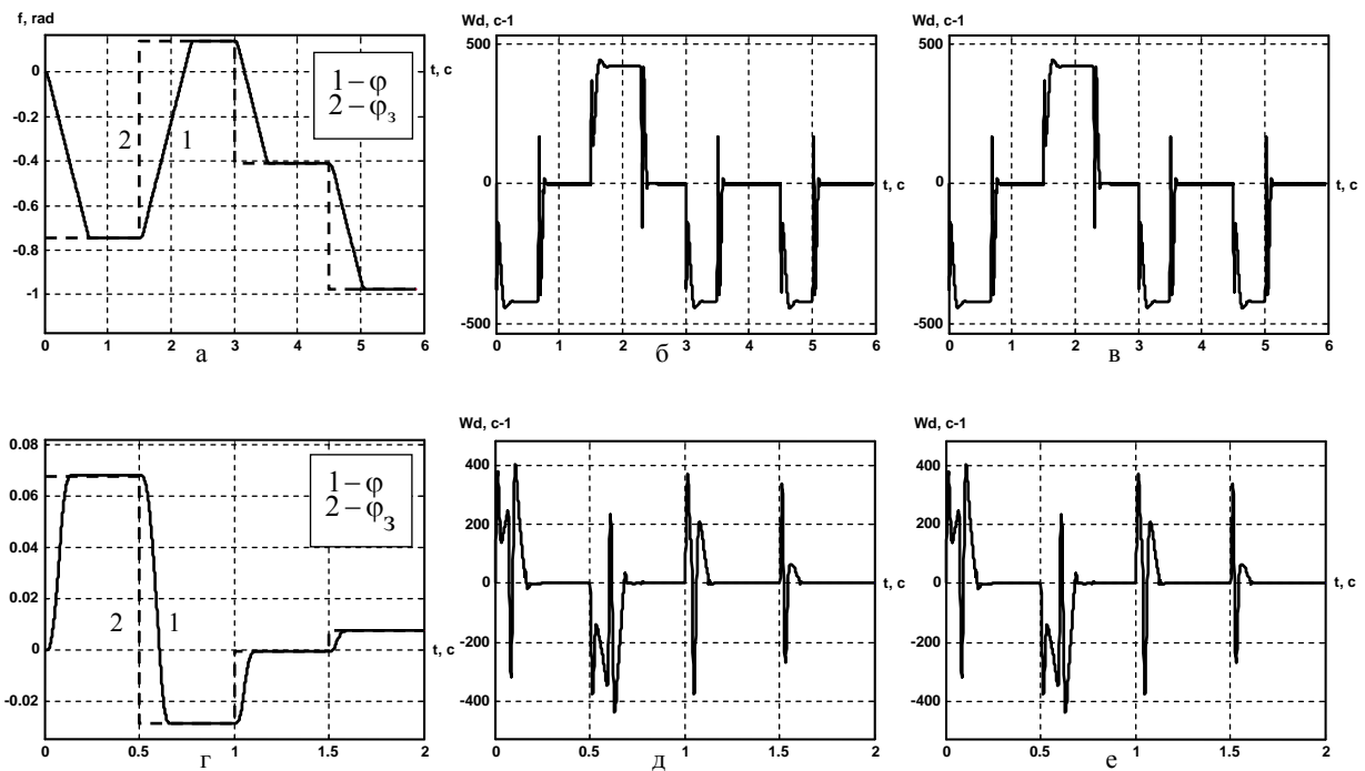
Рис. 4. Графіки перехідних процесів змінних стану системи: а, г – відрізки заданого кута \varphi ; б, д – швидкості механізму \omega_M ; в, е – швидкості двигуна \omega_D
