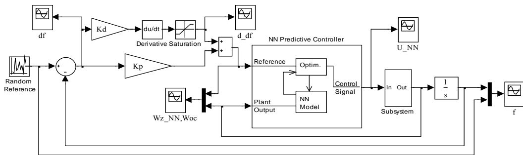
Рис. 1. Схема нейронмережової системи управління
