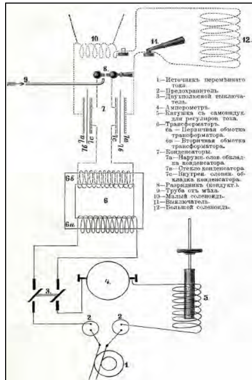
Рис. 7. Схема установки П.И. Ижевского
