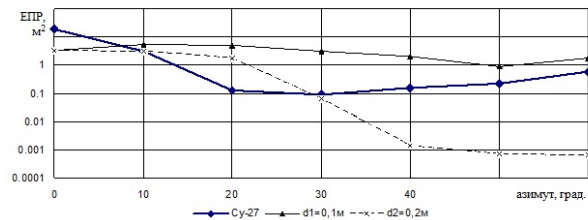
Рис. 5. Залежність медіанних значень ЕПР моделі Су-27і зчтвєреної кутового відбивача з вирізами від азимута опромінення
