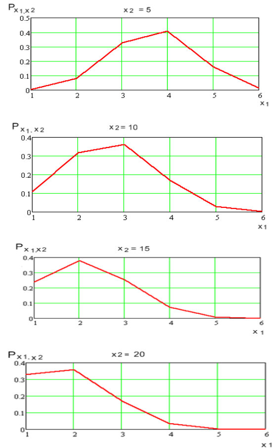
Рис. 3. Графіки функції (8)
