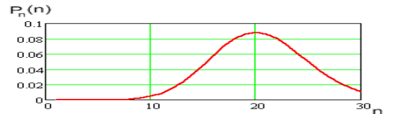
Рис. 2. Графіки функції (7)
