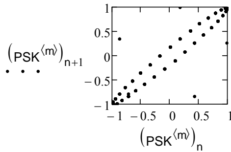
Рис. 3. Фазовий портрет MPSK-сигналу
