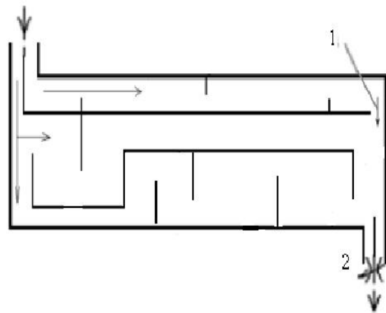
Рис. 4. Схема устрою проточного теплового екрану, який необхідно використовувати: 1 – напрям руху повітря; 2 – регулятор площини перетину вихідного отвору
