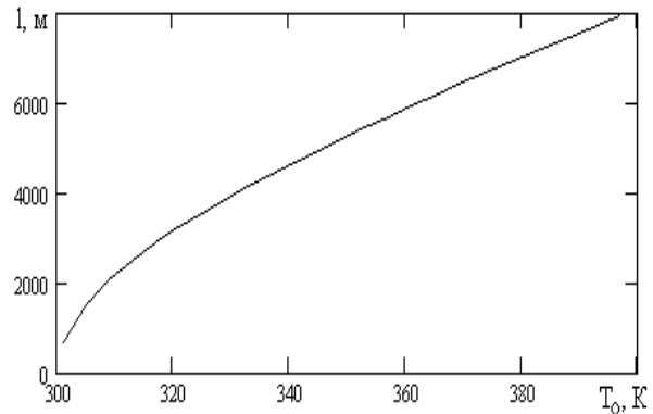
Рис. 3. Залежність відстані, за якої можливе відображення сигнатури об'єкту площею S_o = 10 м 2 у тепловому діапазоні за чутливістю тепловізору \Delta E_{\min} = 1,4 \cdot 10^{-5} Вт/м 2 в залежності від інтегральної температури бронеоб'єкту T_o .
