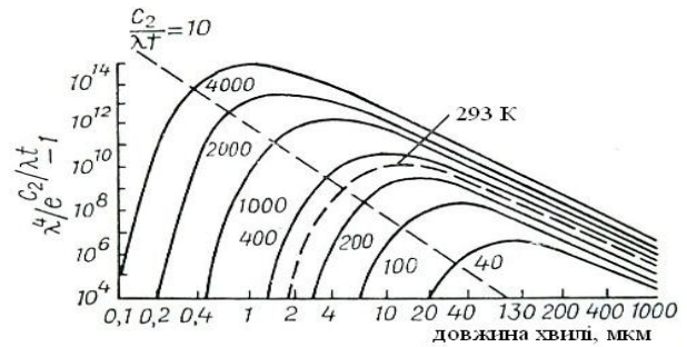
Рис. 1. Ізотерми випромінювання чорних тіл за різною їх температурою, що розраховані за формулою Планка (температура у [K])
